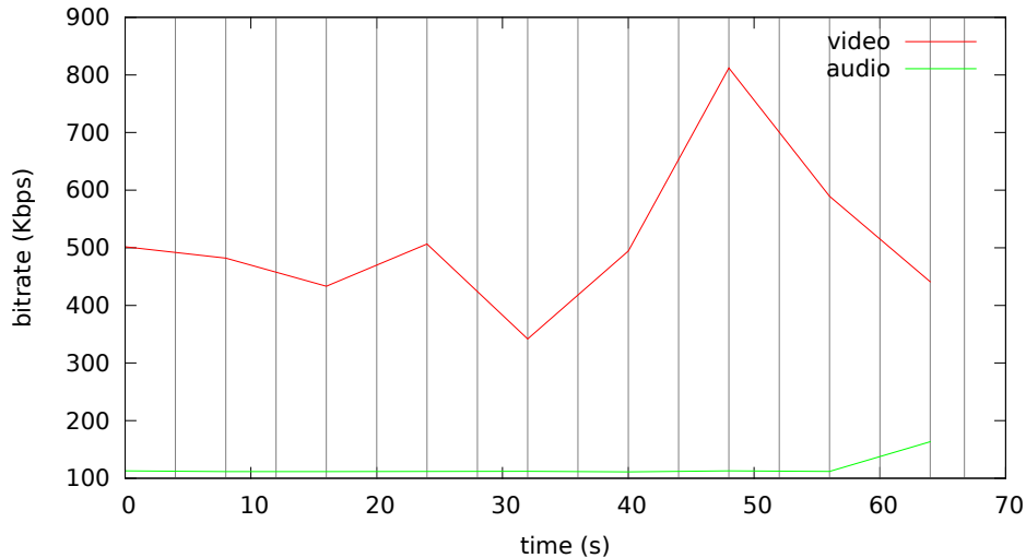
Bitrate analysis of videos-default/fluidmotion-default.mp4
